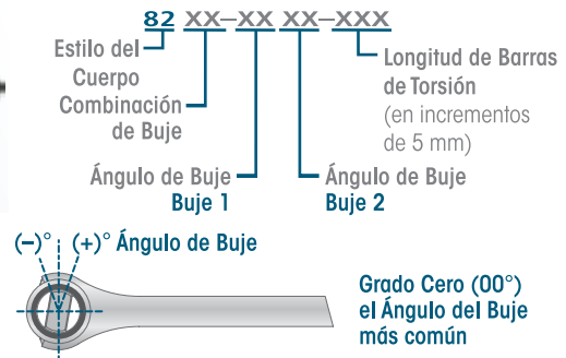
Servicio Pesado – Espárrago / Cónico
